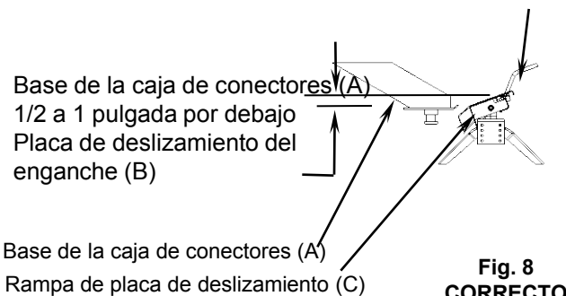
Placa de deslizamiento del enganche (B)
